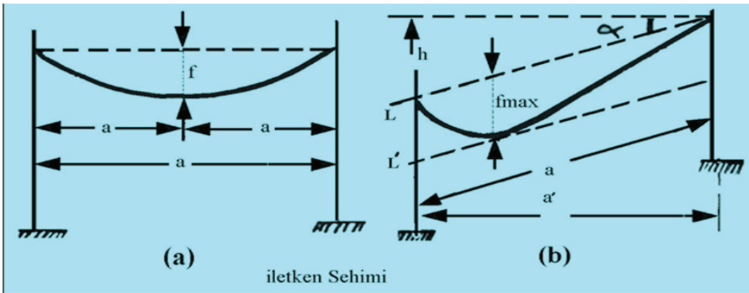
Şekil 13.1 a) Aynı seviyedeki iki direk arasındaki iletkenin sehim b) Seviye (kot) farkı olan iki direk arasındaki iletkenin sehim
