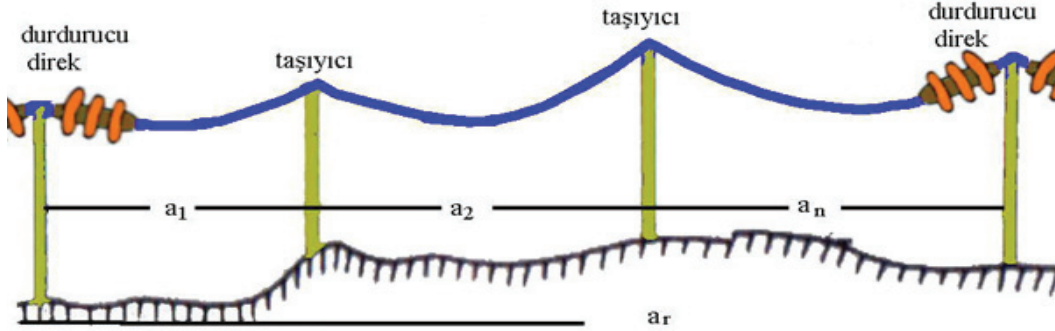
Şekil 13.2 Taşıyıcı, durdurucu direkler ve iletken sehimini
